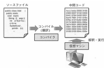
図 7.8 仮想マシンによる中間コードの実行
